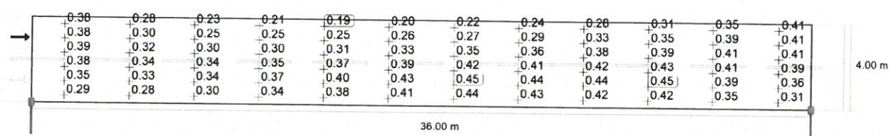
Observator 2: Valoarea de întreținere, densitatea luminii cu carosabil uscat [ \text{cd/m}^2 ] (Raster valoric)
