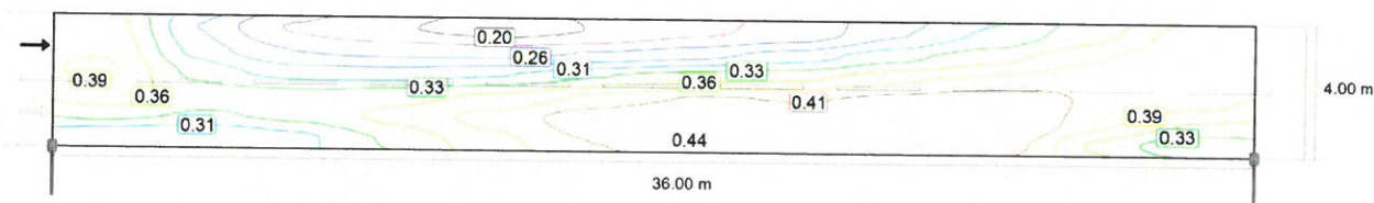
Observator 2: Valoarea de întreținere, densitatea luminii cu carosabil uscat [ \text{cd/m}^2 ] (Linii Isolux)
