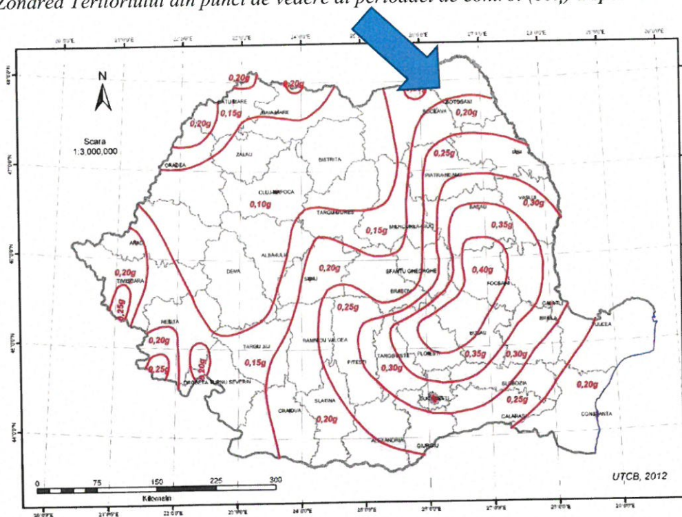
Fig.6 – Zonarea accelerației terenului
